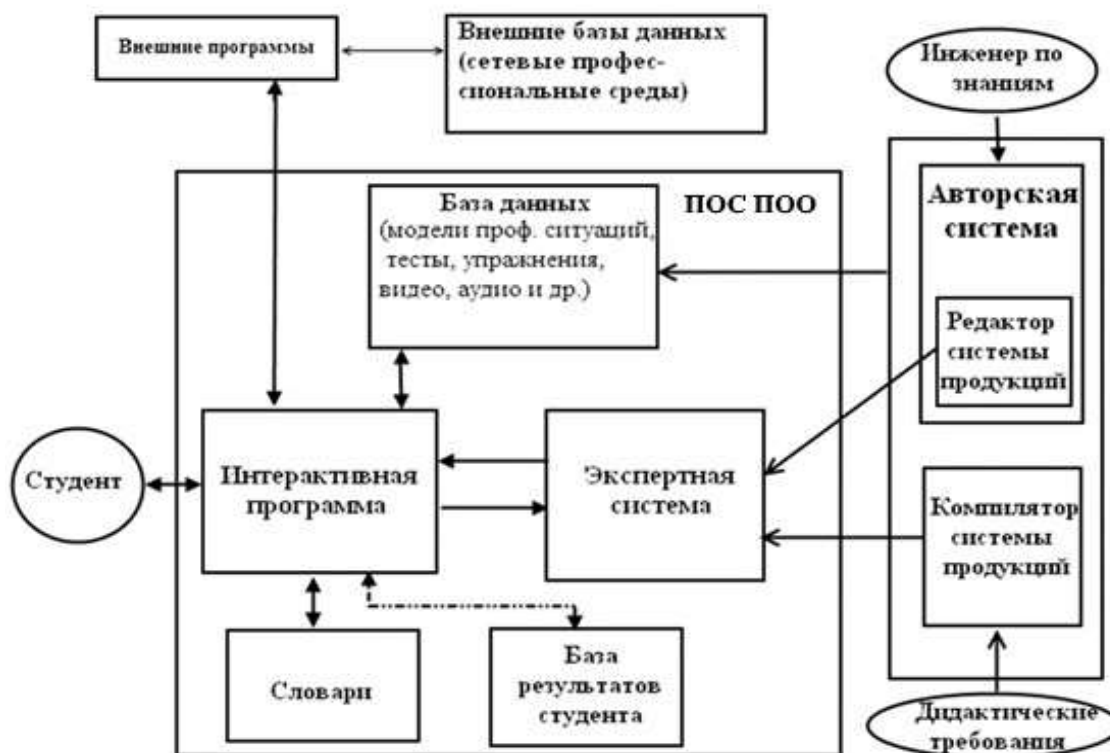
Рис. 1. Структурная схема экспертной системы, адаптированной для ПОС ПОО
